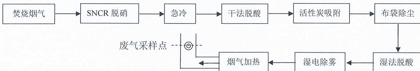
废气处理工艺流程图
